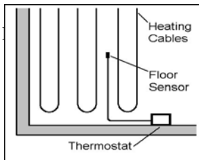
Рис. 1: Установка датчика температуры пола
